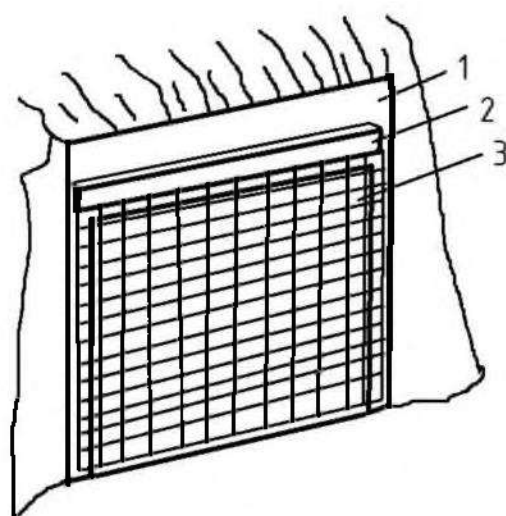
1-портал людского вход в сооружение; 2-конструкция крепления «висячей шторы»; 3-«висячая штора»
