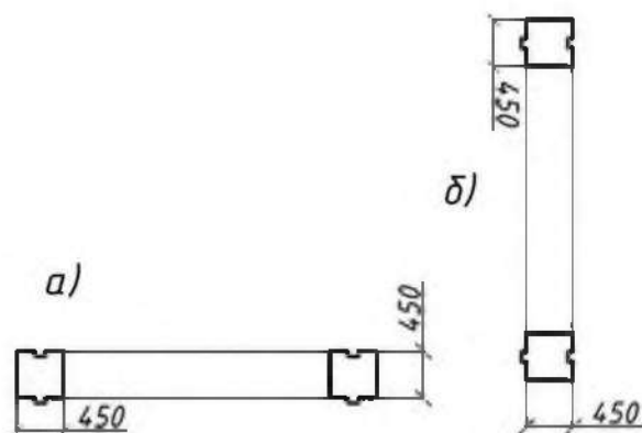
а – горизонтальный элемент; б – вертикальный элемент
