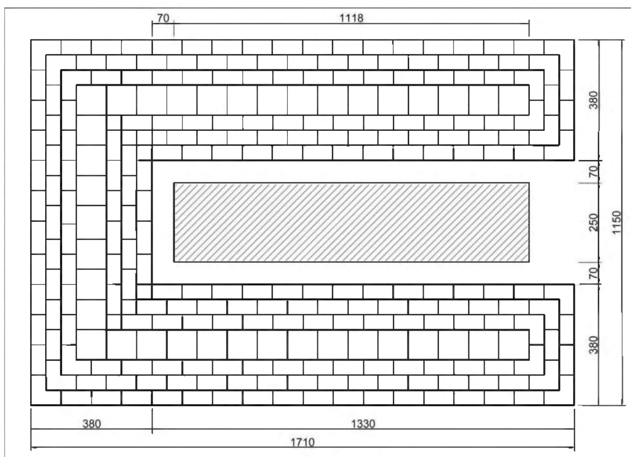
Рисунок V.56 - План укрытия окопа - укрытия ракетно-пушечной установки «Панцирь-С1» с применение мягких контейнеров типа «БИГ-БЭГИ», установленных в четыре яруса
