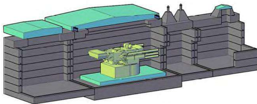
Рисунок V.43 - Комплекс ПВО «Панцирь – Ф» в сборном варианте из горизонтальных рам
