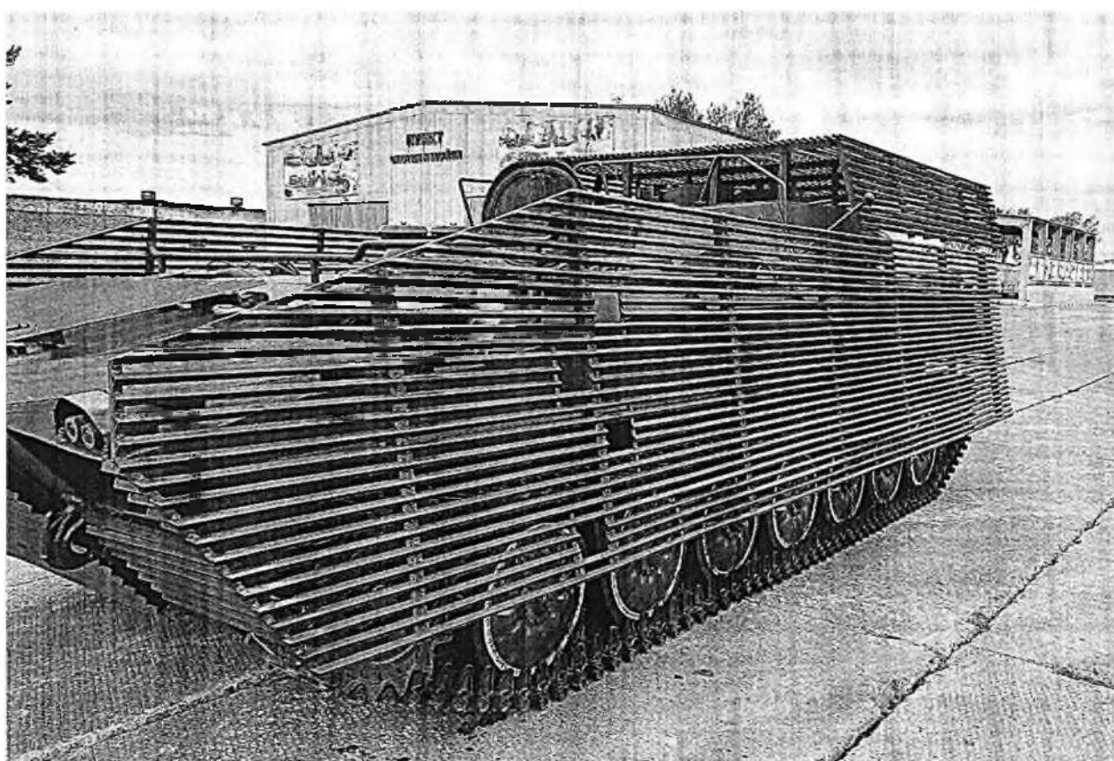
Рисунок III.6 - Пример защиты УР-77. Вид с левого борта
