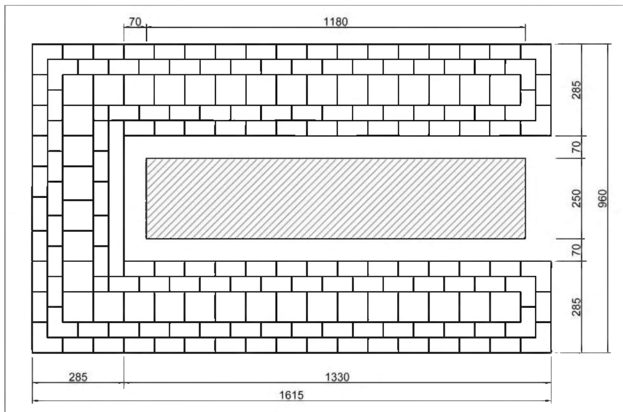
Рисунок V.53 - План окопа - укрытия для ракетно-пушечной установки «Панцрь-С1» с применение мягких контейнеров типа «БИГ-БЭГИ», установленных в три яруса
