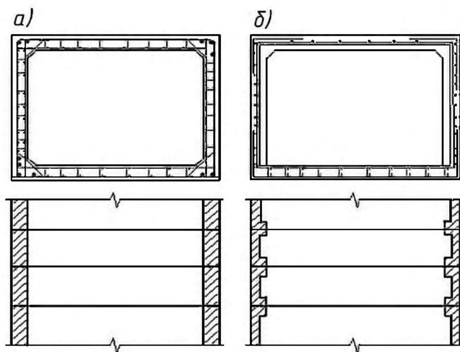
a – прямоугольного сечения; б – ребристых
