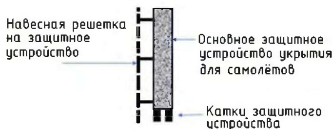
Рисунок V.72 – Навесная решётка на ворота укрытия самолёта
