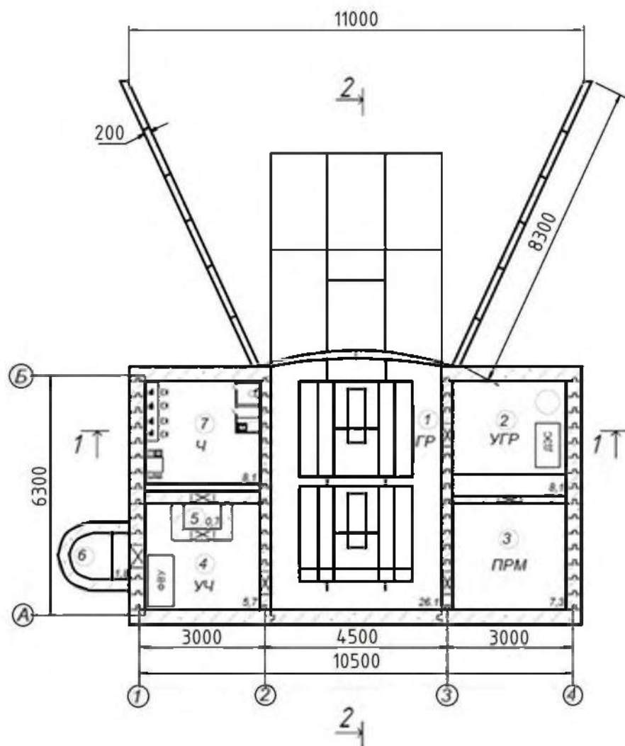
Рисунок V.82 - Принципиальная схема СФС для защиты БЛС. План
