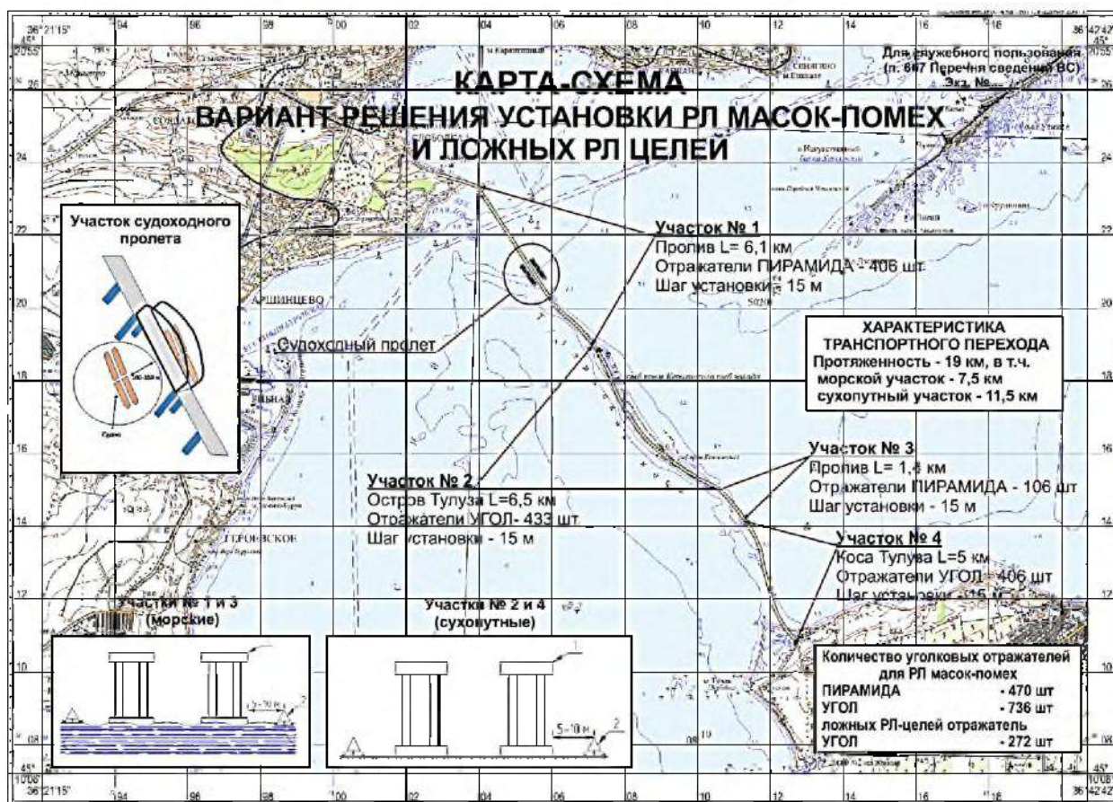
Рисунок III.44 – Карта-схема. Вариант решения установки РЛ масок-помех и ложных РЛ целей
