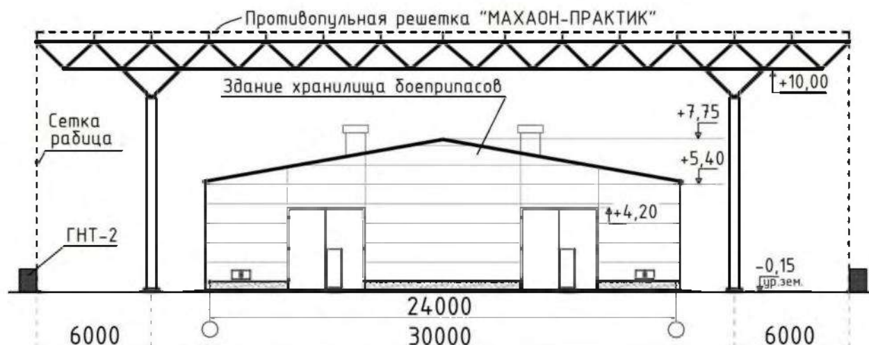
Рисунок IV.31– Схема защиты здания хранилища боеприпасов с использованием структурного покрытия с дополнительной защитой противопоульной сеткой «МАХАОН-ПРАКТИК» и сетки рабица
