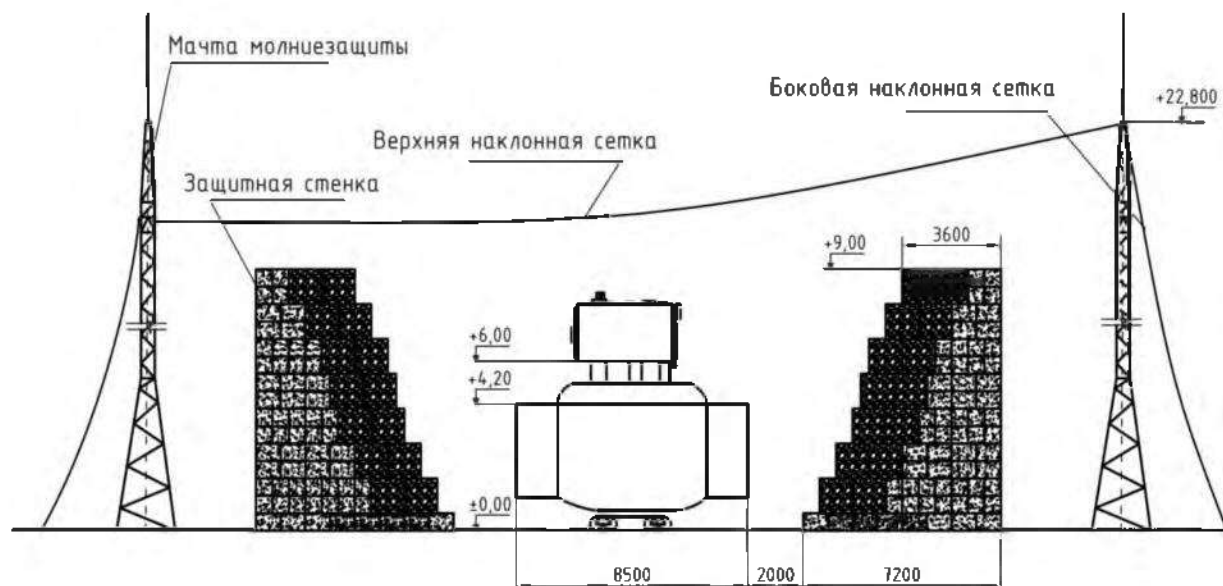
Рисунок IV.5 - Техническое предложение по защите силовых трансформаторов от ударов БПЛА типа «Баба-Яга» и 155-мм снарядов артиллерии ВСУ
