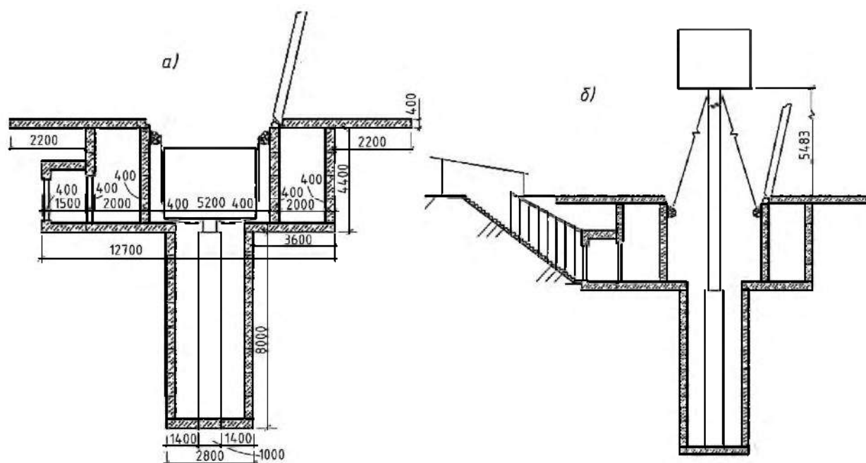
а) крышка открыта; б) крышка открыта, антенна в боевом положении Рисунок V.28 – Разрез защищённого командного пункта ЗРК
