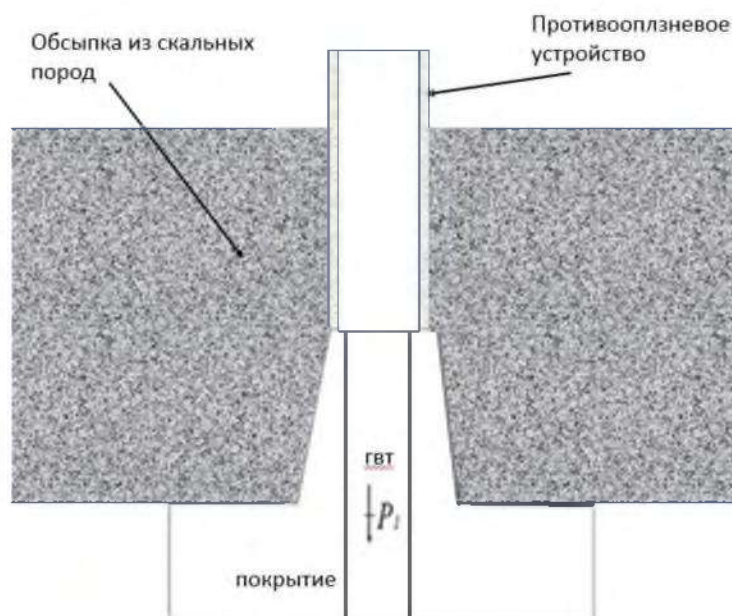
Рисунок V.68 – Тюфяк СФС из скальных пород с противооползневым устройством
