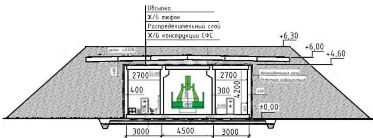
Рисунок V.83 - Принципиальная схема СФС для защиты БЛС. Разрез 1-1
