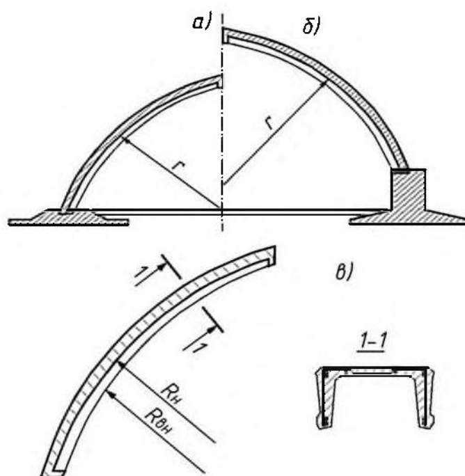
a, б – круглое очертание арки; в – стрельчатая панель и разрез панели
