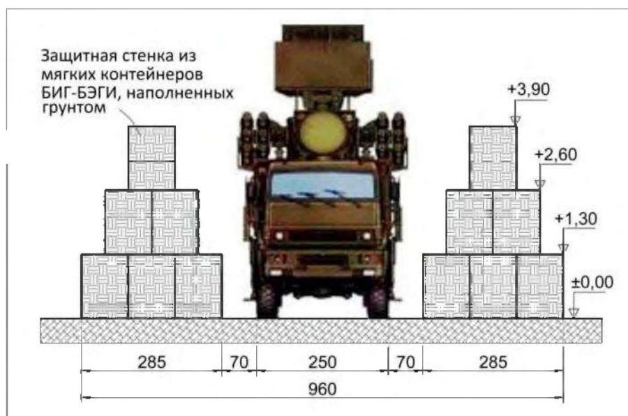
Рисунок V.55 - Поперечный разрез окопа - укрытия для ракетно-пушечной установки «Панцирь-С1» с применение мягких контейнеров типа «БИГ-БЭГИ», установленных в три яруса
