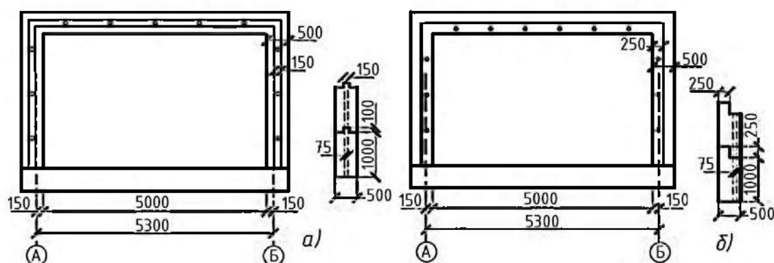
a – в шпунт; б – в четверть
